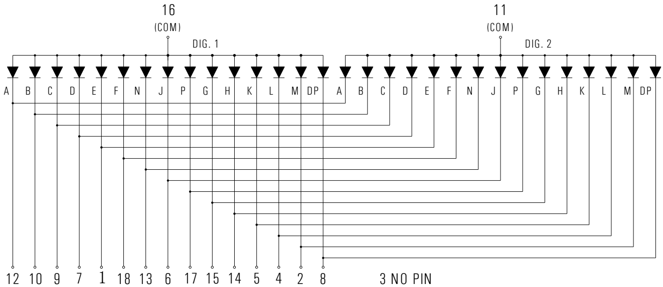
KA2-541ABB (Common Anode)
