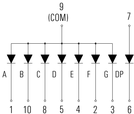
KD1-321AYD-2B (Common Anode)
