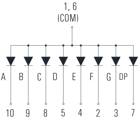
KD1-40NAYD-2B (Common Anode)
