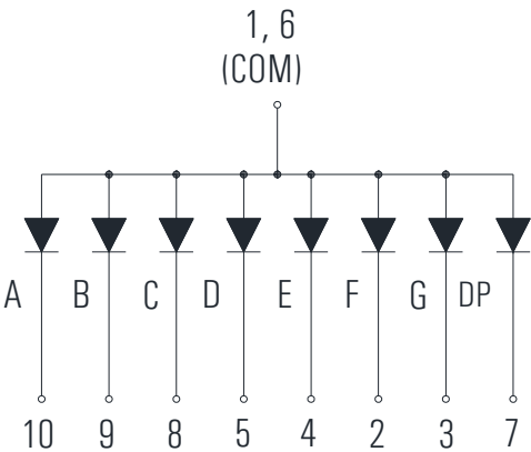
KD1-40NAYD-3C (Common Anode)
