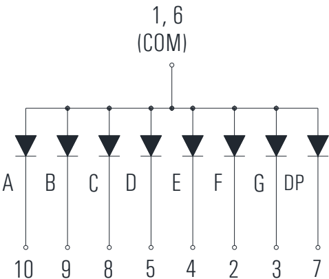
KD1-40NAGD-2B (Common Anode)
