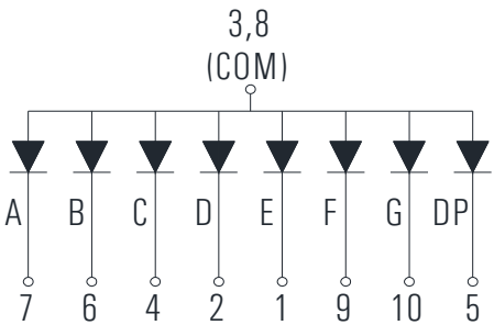
KD1-501ARB-08C30 (Common Anode)
