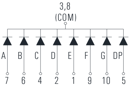
KD1-501CRB-08C30 (Common Cathode)
