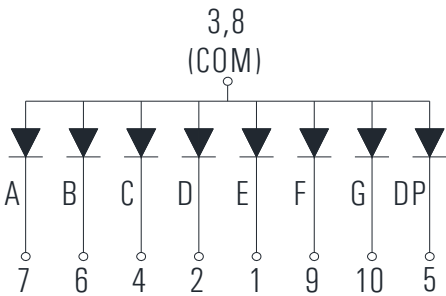
KD1-571AGD-2B (Common Anode)
