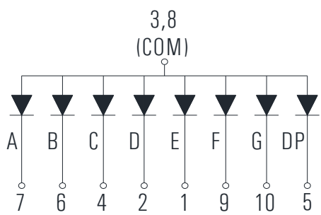
KD1-571AYD-2B (Common Anode)
