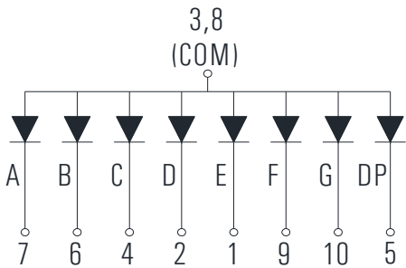
KD1-571AYD-3C (Common Anode)
