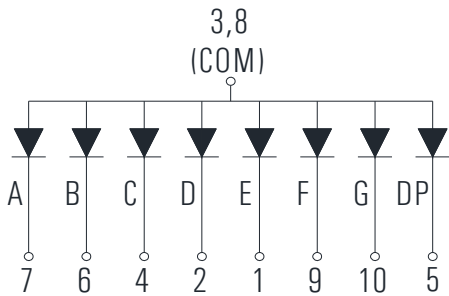
KD1-571AAD-2B (Common Anode)
