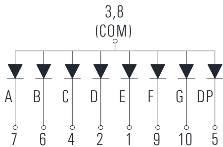
KD1-571AVD-2B (Common Anode)
