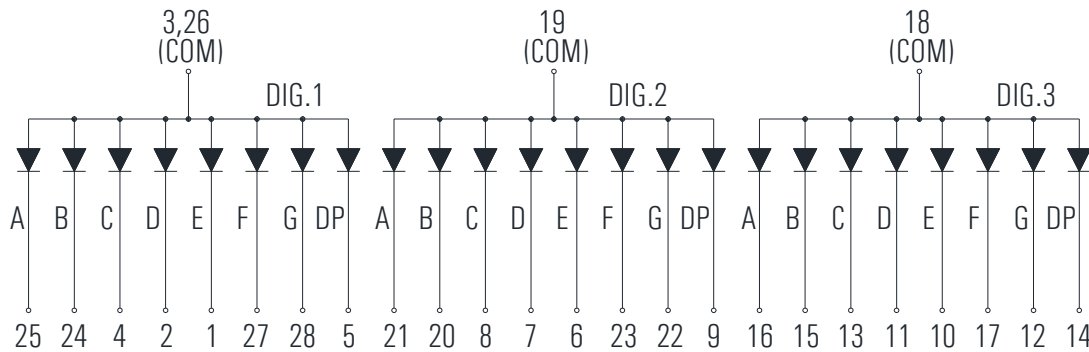
KD3-56BARD-S (Common Anode)
