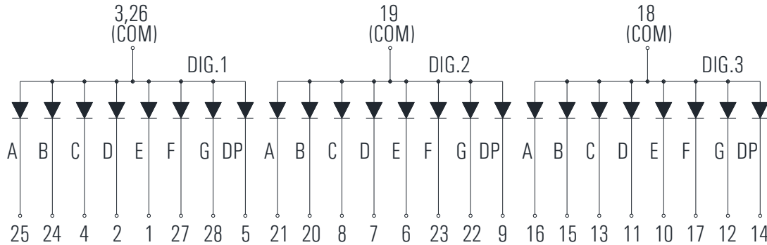
KD3-56BAGD-S (Common Anode)
