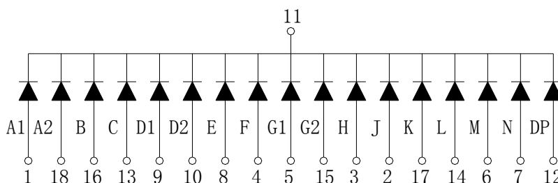
KWA-801CGA
