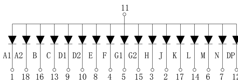
KWA-801AGA
